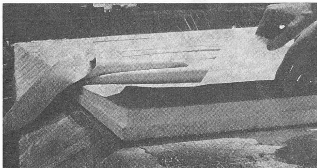
Oberer Abschluss des Eisfeldes; über der Dampfsperre eine Hart-schaumisulationsplatte von 5 cm Stärke, die den dünnen Kieskoffer kompensiert. Es folgen: eine Gleitschicht, PVC-Folie als Wasserisolation, darüber Schutzmörtel und armierte Betonplatte mit Kühlrohren
