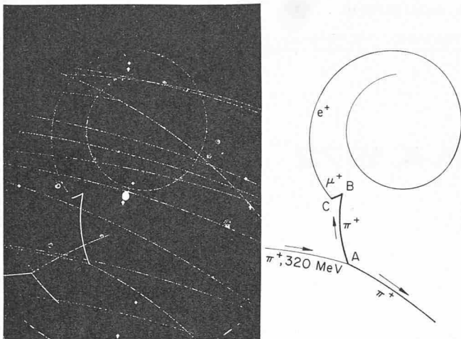
Bild 2. Erzeugung und Zerfall eines \pi^+ -Mesons im flüssigen Wasserstoff einer Blasenkammer des CERN. Das von links einfallende \pi^+ -Meson stösst bei A auf ein Proton des flüssigen Wasserstoffes. Das Proton wird dabei in ein Neutron verwandelt, und es entsteht aus übriggebliebener Energie ein weiteres, elektrisch positiv geladenes \pi^+ -Meson, das von A nach B fliegt. Auf seinem Flug durch die Flüssigkeit wird es ständig gebremst. Bei B kommt es zur Ruhe. Im Mittel nach 2,6 \cdot 10^{-8} s zerfällt es in ein positiv geladenes Müon ( \mu^+ ) und ein Neutrino. Das Neutrino hinterlässt in der Blasenkammer keine Spur, da es elektrisch ungeladen ist. Das \mu^+ fliegt von B nach C und kommt dort zur Ruhe. Nach 2,2 \cdot 10^{-6} s zerfällt es in ein Positron e^+ (= positives Elektron) und zwei (nicht sichtbare) Neutrinos. Das Positron beschreibt im Magnetfeld der Blasenkammer eine Kreisbahn, deren Radius wegen der Bremsung in der Flüssigkeit ständig abnimmt (Photo CERN)
