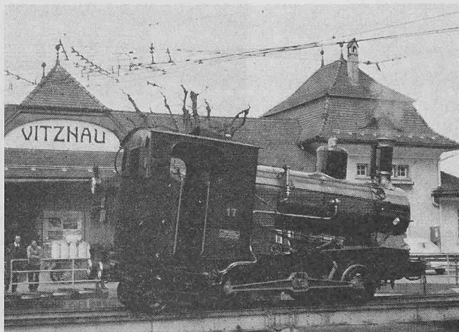
Bild 6. Dampflokomotive mit liegendem Kessel, Fabrikat SLM (heute noch betriebsbereit)
