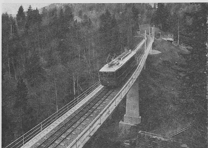
Bild 5. Neue Schnurtobelbrücke aus Spannbeton
