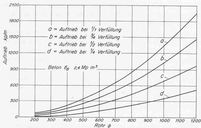
Bild 4. Auftriebswerte von Hohlkörpern mit rundem Querschnitt in Beton von 2,4 t/m³
