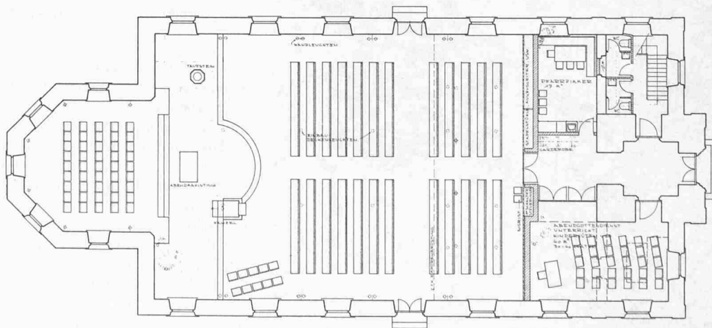
Bild 20. Kirche Wil. Grundriss 1 : 300. Renovationsprojekt 1969 von Werner Blumer (Zollikon). Turmseitig vorgeschobene Schiffs-Rückwand, dahinter neues Pfarrzimmer und neuer Unterrichtsraum. Reduzierte mobile Bestuhlung (auch im Chor). Neue Orgel-empore; Decke tiefer gehängt (nicht ausgeführt)
