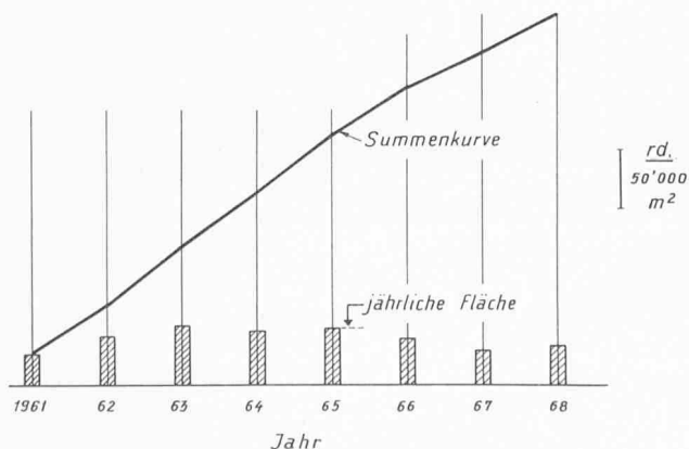
Bild 6. Herstellung von Schlitzwänden in der Schweiz, 1961 bis 1968 (Schätzung)
