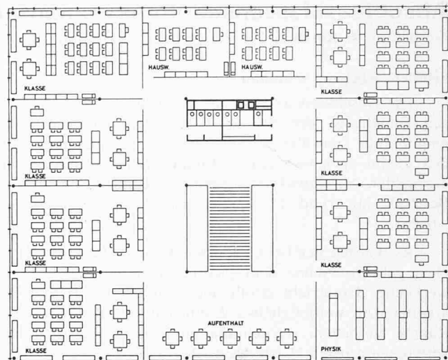
Schulhaus. Normalgrundriss 1:400
