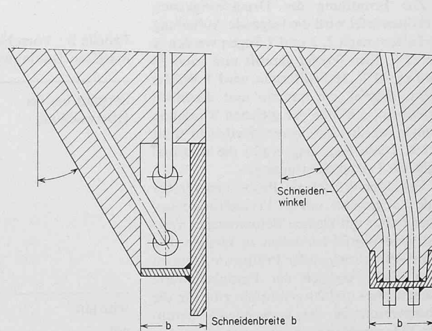
Bild 2. Schachtschneiden und ihre Panzerung
