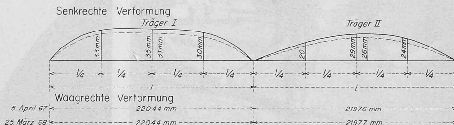
Bild 6. Verformung der Träger nach einem Jahr unter p = 0,3 \text{ t/m}^2 Nutzlast
