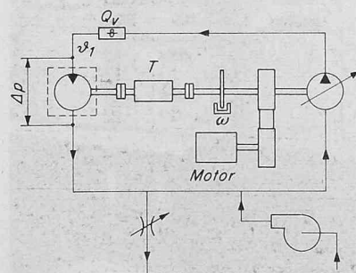
Bild 33. Anordnung mit einer Hydromotor als Belastung. Diese entspricht der in Bild 30 gezeigten, mit dem Unterschied, dass hier am Hydromotor gemessen wird
