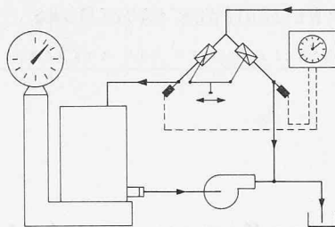
Bild 2. Messung mittels Wägung; Zeitmessung mit Stoppuhr
