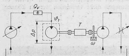
Bild 33. Anordnung mit einer Hydromotor als Belastung. Diese entspricht der in Bild 30 gezeigten, mit dem Unterschied, dass hier am Hydromotor gemessen wird
