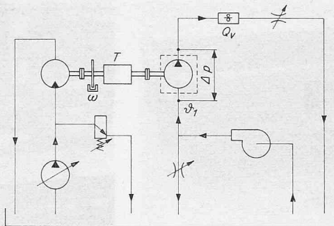
Bild 30. Hydromotorantrieb. Die für den Versuch benötigte Energie wird von einem Hydromotor geliefert. Die Drehzahleinstellung erfolgt durch Änderung des Hubvolumens einer hydraulischen Pumpe, die Druckeinstellung durch einen verstellbaren hydraulischen Widerstand
