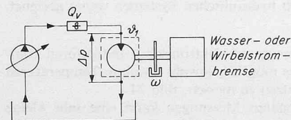
Bild 32. Pendelanordnung mit einer verstellbaren Hydromotor. Die gesamte Energie wird von der Hydromotor geliefert. Die Drehzahleinstellung erfolgt durch Änderung des Pumpenhubes, die Druckeinstellung wird mit der Wasserbremse vorgenommen. Da die Wasserbremse pendelnd aufgehängt ist, erfolgt eine Messung des Reaktionsmoments
