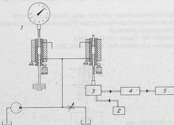
Bild 15. Schema einer Messeinrichtung mit Kolbenmanometer 1 Eichereinrichtung, 2 Spannungsquelle, 3 Kraftmessdose, 4 Verstärker, 5 Anzeige
