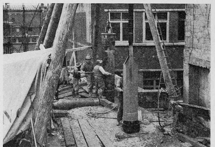
Bild 9. Herstellung von Bohrpfählen mit einfachem Dreibein und Bohrwerkzeug
