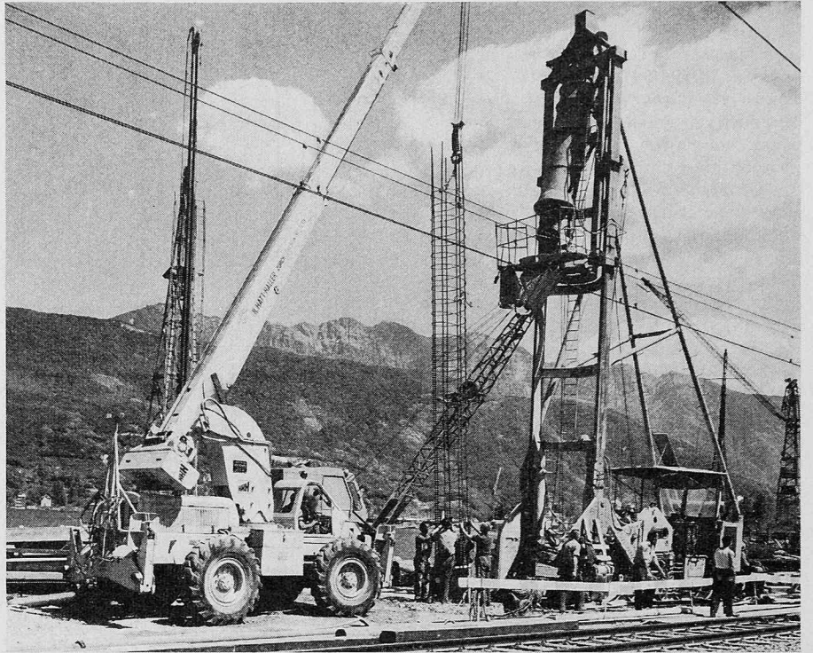
Bild 7. Benoto-Maschine (Schlagbohrverfahren)
