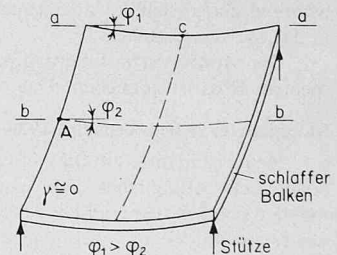
Bild 3. Quadratplatte auf schlaffen Randbalken (Vierpunktstützung) allseitig aufgelagert ( \gamma \approx 0 )
