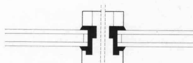
Ciba AG, Laborhochhaus, Basel Architekten: Suter & Suter, Basel Verglasung: ISAL, Hans Schmidlin AG, Aesch-Base
