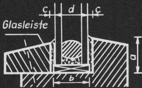
Je nach Anwendungsgebiet können Rahmen aus Holz, Stahl, Leichtmetall, Kunststoffen oder Beton Verwendung finden.
