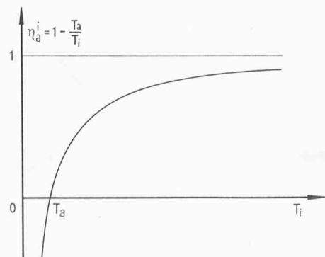
Bild 3.2. Carnotwirkungsgrad \eta_a^i in Funktion der Temperatur T_i , mit welcher die Wärme von der Wärmequelle i aufgenommen wird
