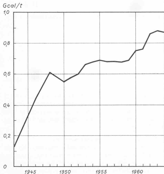
Bild 1. Entwicklung der spezifischen Wärmeproduktion in Gcal/t Kehrriecht der KVA Basel
