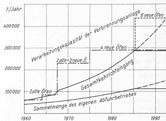
Bild 3. KVA Basel: voraussichtliche Entwicklung der Kehrrichtmengen für Verbrennung und Abfuhr und der Verarbeitungskapazität der Verbrennungsanlagen
