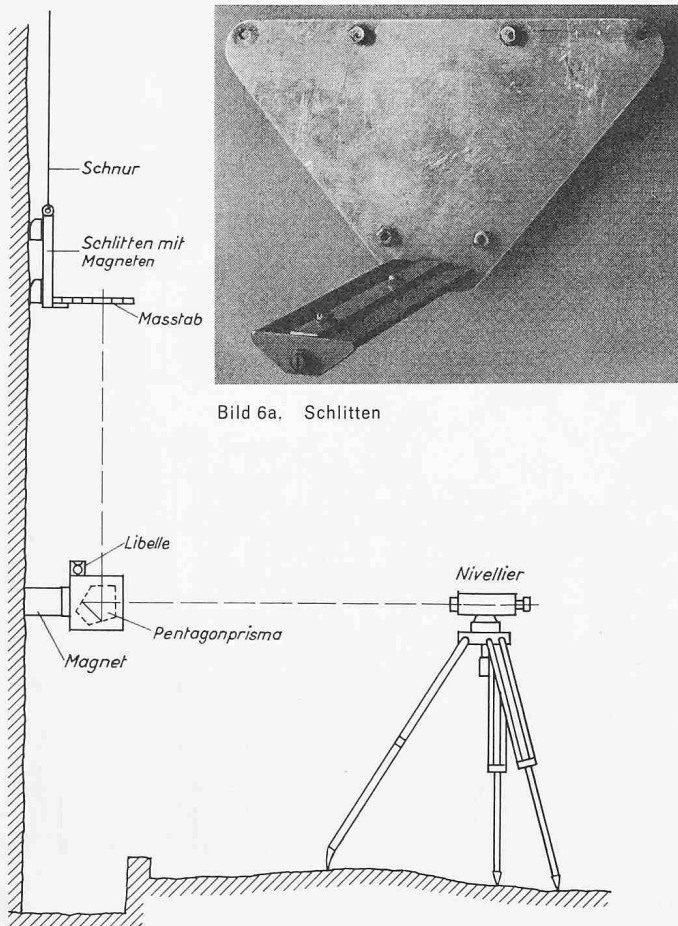
Bild 6. Optische Ablotung
