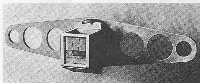
Bild 8. Pentagon-Prisma mit Libelle und Griffen zur Justierung
