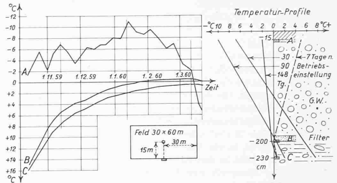
Bild 8. Kunsteisbahn Uzwil, Winter 59/60
