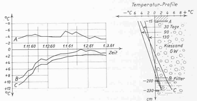
Bild 9. Kunsteisbahn Uzwil, Winter 60/61
