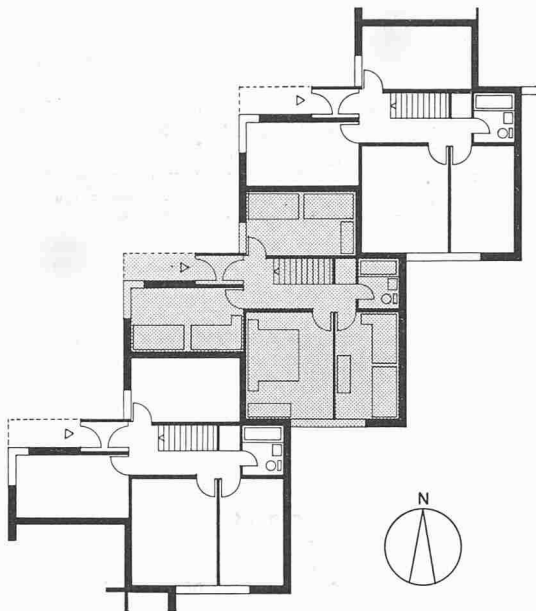
Reihenfamilienhäuser R, Fünfzimmerhaus 1:300 Eingangsgeschoss
