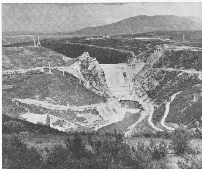
Wasserkraftanlagen Bárceña der Servicios Hidráulicos del Norte de España, Mauerhöhe 109 m, installierte Leistung 2x18 000 kVA
