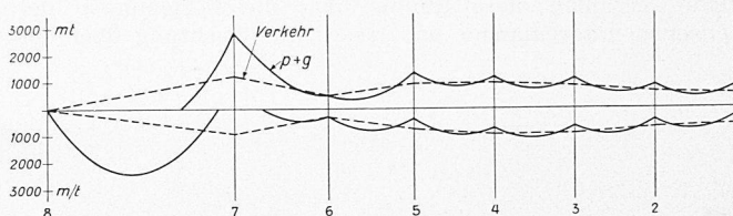
Bild 8. Momentengrenzerte der Fahrbahn
