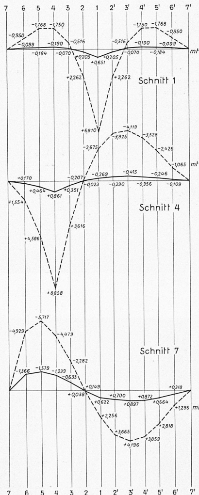
Bild 8. Momentengrenzerte der Fahrbahn
