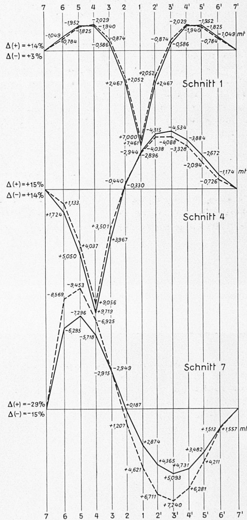
Bild 8. Momentengrenzerte der Fahrbahn
