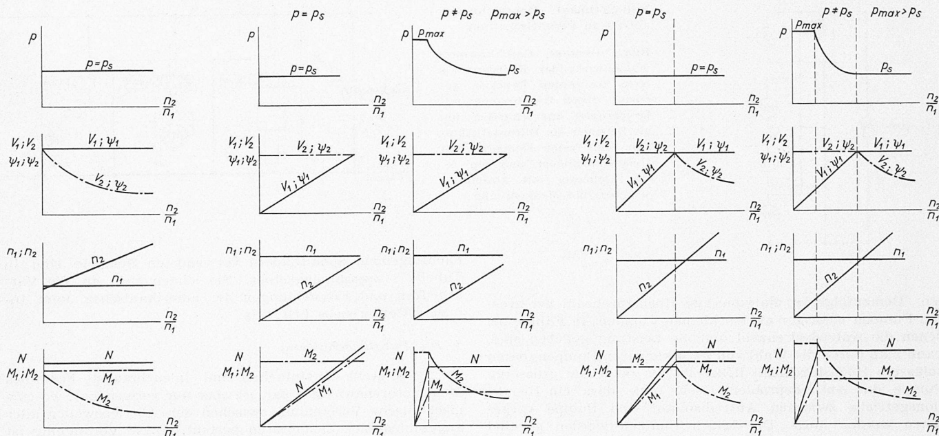
Bild 9. Sekundärregulierung
