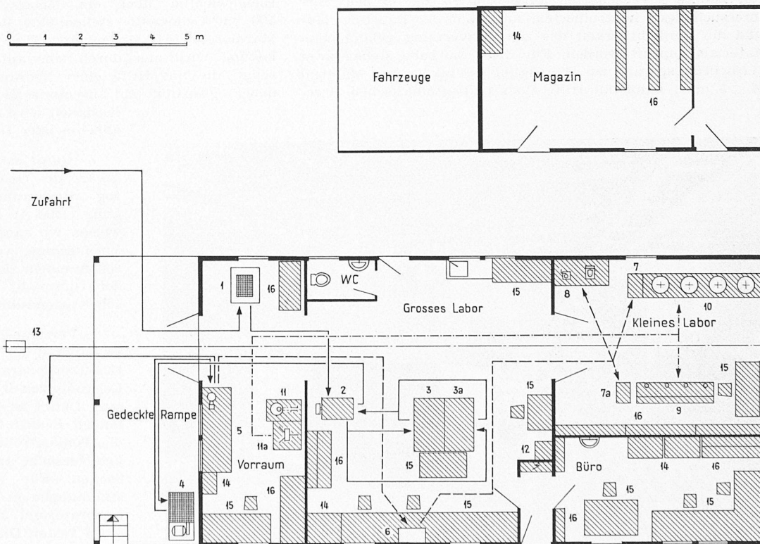
Bild 4. Grundriss des Feldlaboratoriums, Masstab 1:150
