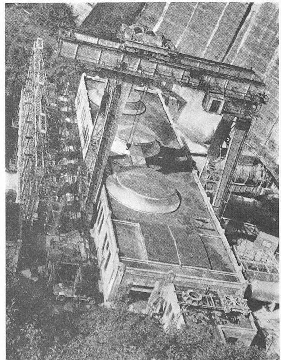
Bild 11 (links). Merwin-Bogenmauer von der Luftseite
