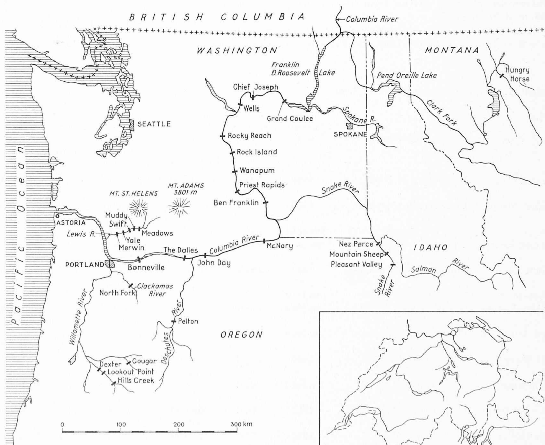
Bild 1. Ubersichtsplan der Wasserkraftanlagen im Northwest Power Pool, USA. Rechts die Schweiz im gleichen Masstab, 1:6 500 000 (Länge des Columbia River 2000 km, des Rheins 1300 km)
