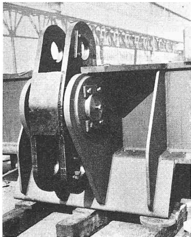
Bild 5. Aufhängung
