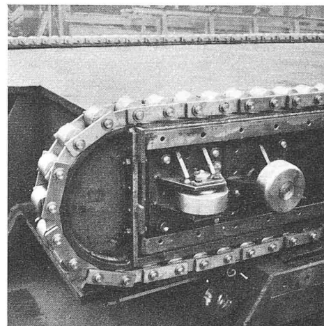
Bild 7. Führungsräder
