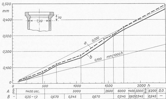
Bild 11. Durchmesserergrößerungen eines Zylindereinsatzes von 720 mm Bohrung und 1250 mm Hub infolge Abnutzung im Verlaufe von rd. 2500 Betriebsstunden mit verschiedenen Brennstoffen mit Viskositäten zwischen 1400 und 6200 sec. Redwood I, gemessen mit pneumatischem Gerät; a) Mittelwert der Messungen senkrecht und parallel zur Motorlängsachse, b) Mittelwert von 24 Messstellen am Umfang, A Viskosität des Brennöls in sec. Red. I/100 ° F (DO = Dieselöl) B Zentrifugendurchsatz in t/h
