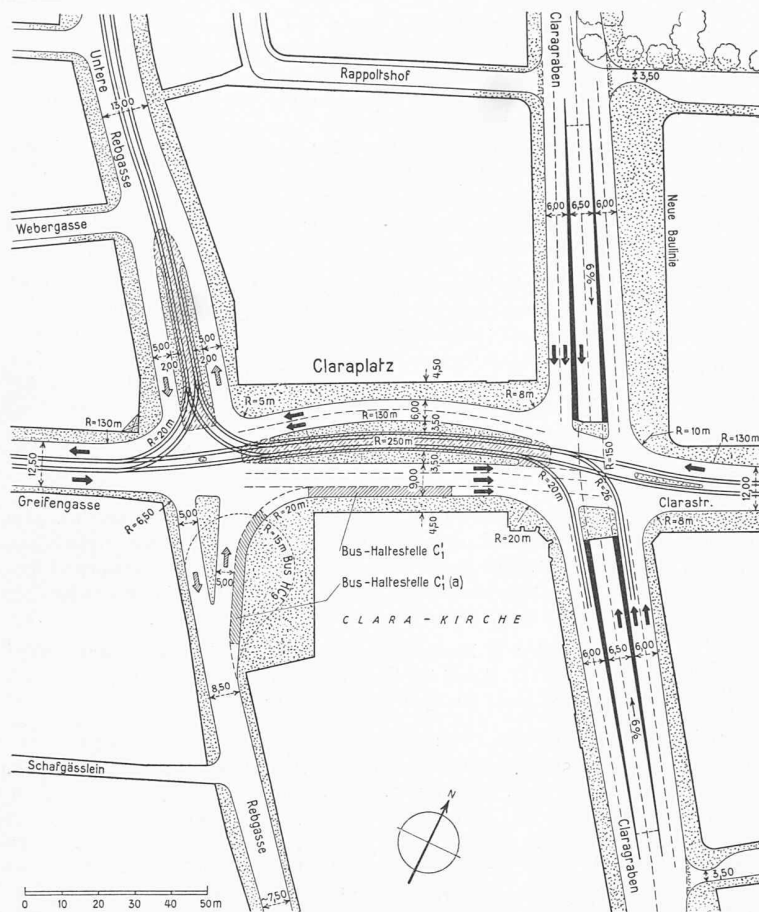
Bild 8. Vorschlag für die bauliche Gestaltung des Claraplatzes in Basel Massstab 1:2000
