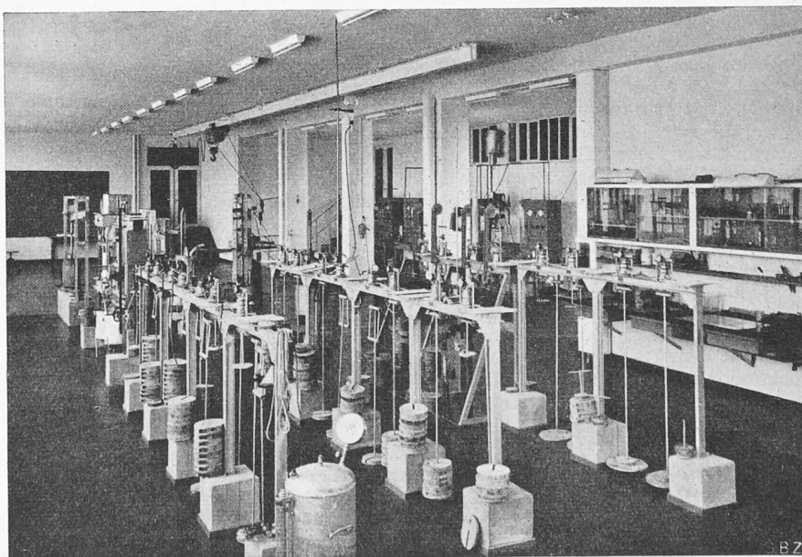
Bild 4. Blick in das Hauptlaboratorium der Erdbauabteilung mit Zusammendrückungsapparaten (vorn) und grossem Triaxialapparat (hinten, rechts)
