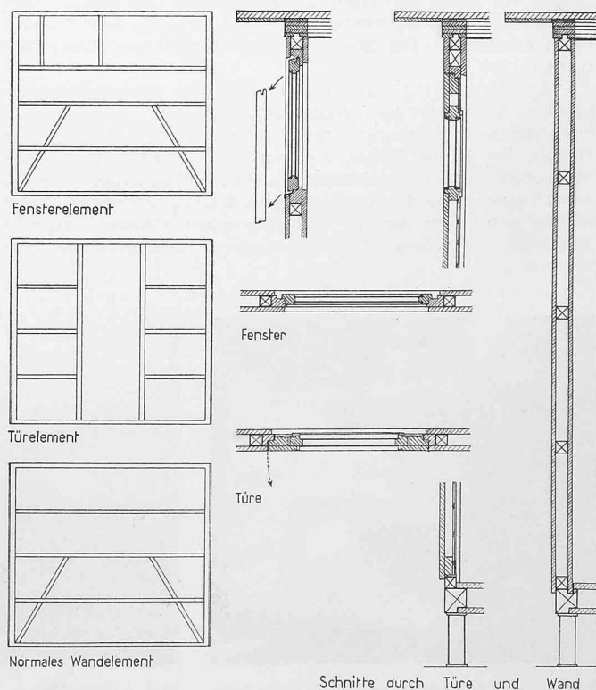
Bild 11. Wandelemente 1:75, Schnitte 1:25
