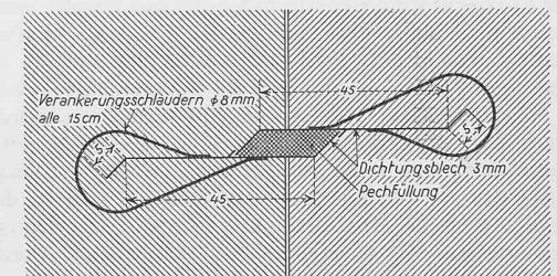
Bild 9. Mauerfugen-Dichtung, Horizontalschnitt 1:15
