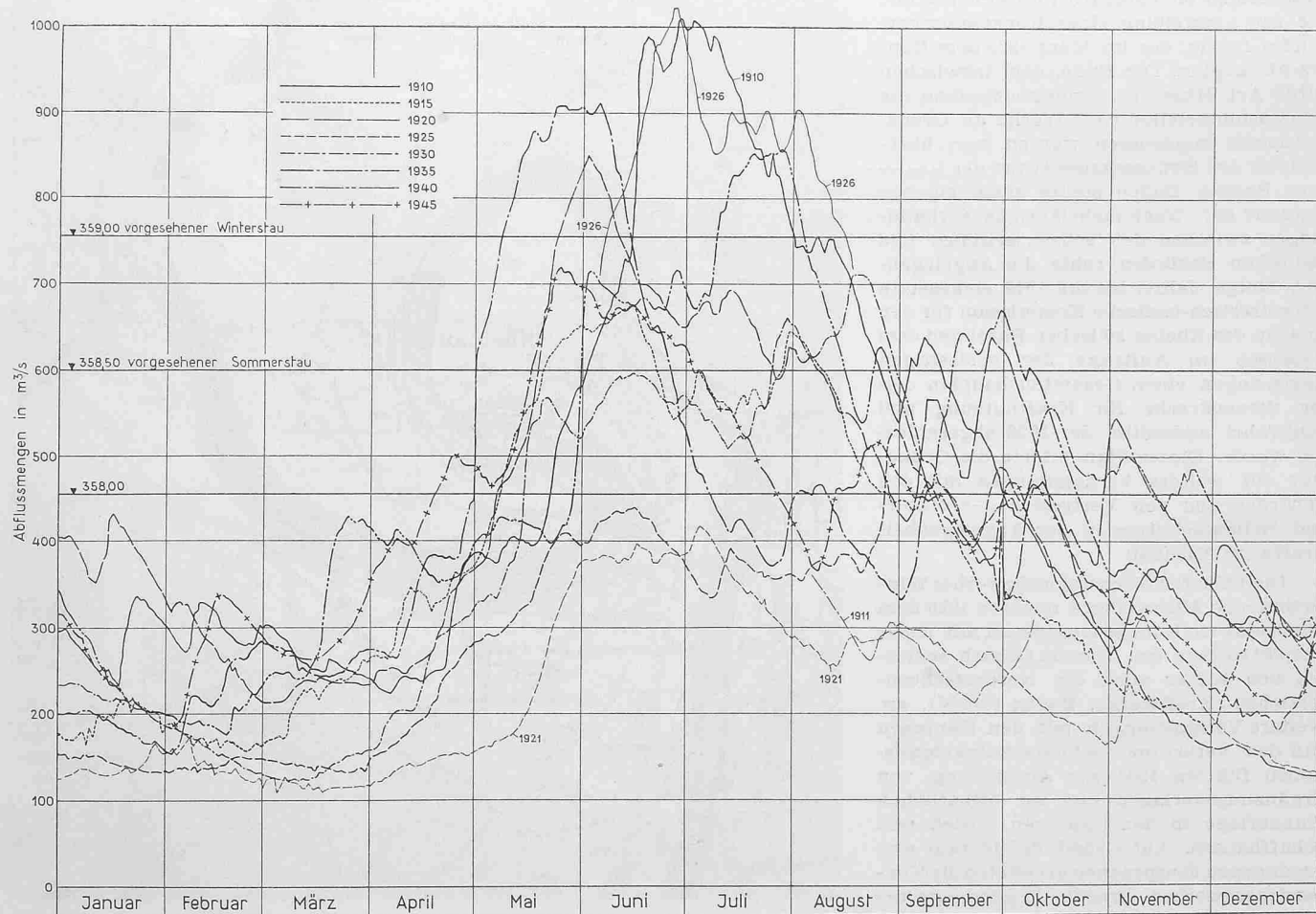
Bild 3. Natürliche Wasserspiegelschwankungen im Rheinflallbecken in der Zeit von 1910 bis 1945 (alle fünf Jahre, sowie in den extremen Perioden der Jahre 1911, 1921 und 1926)
