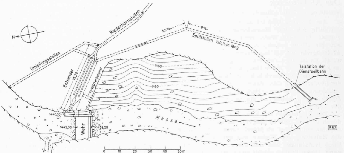
Bild 4. Wasserfassung des Aletschwerkes, Masstab 1 : 1500
