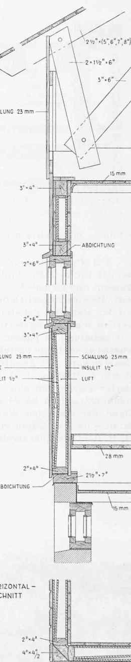
Bild 2. Konstruktion des Hauses Bild 1, Masstab 1:25
