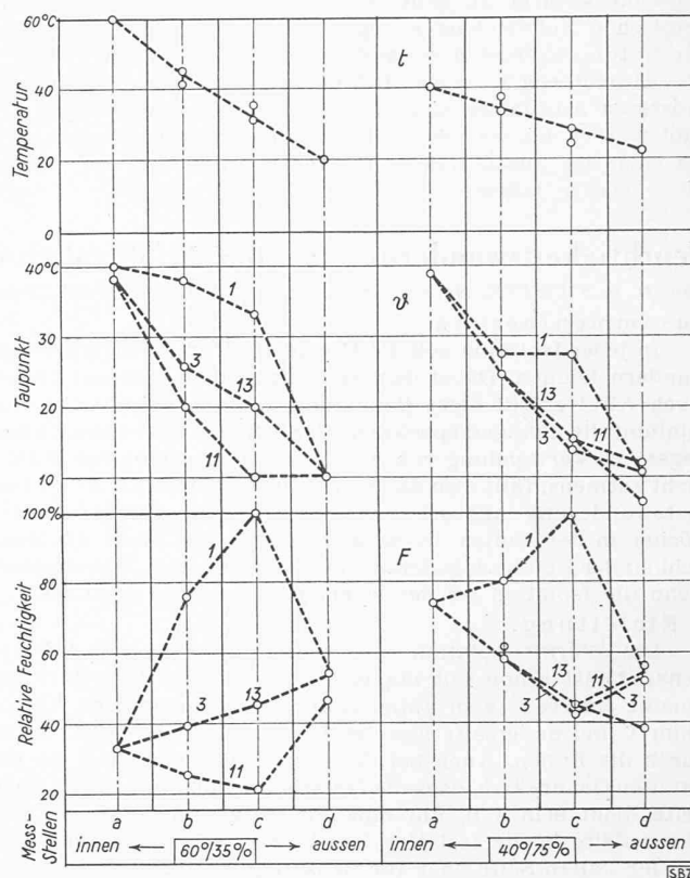
Bild 4. Temperatur t , Taupunkt \phi und relative Feuchtigkeit F in Isolationsschichten von je drei gleichen Folien. Hohe Feuchtigkeitswerte (Nummern der Folien siehe Tabelle 1)
