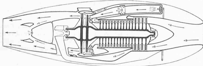
Bild 10. Prinzipskizze des Doppelstromtriebwerkes Rateau-Anxionnaz SRA-1
