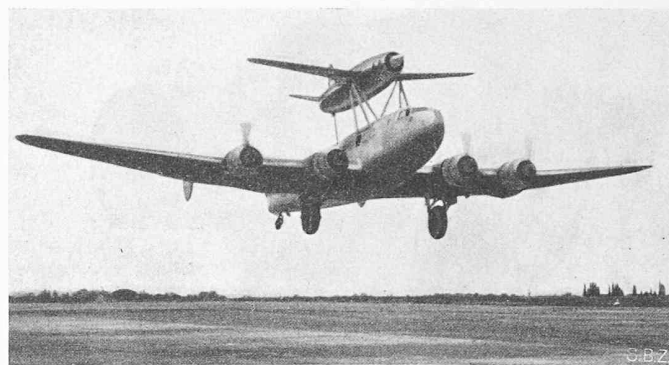
Bild 13. Flugzeug «Leduc 010» mit Thermo-Düsenantrieb. Versuchsflug mit einem viermotorigen Mutterflugzeug «Languedoc»
