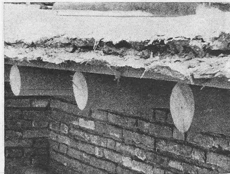
Abb. 13. Bungalow des Obersten Mohamed Arif Khan, Kabul (E. A. Engler, Arch. S.I.A.). Traufkante des Lehmhauses während d. Herstellung
