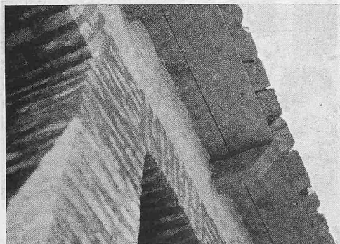
Abb. 12. Kleine Soldatenmoschee (Baubureau Armeekorps Kabul). Lehmhaus mit Traufkante aus Steinplatten
