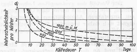
Abb. 4. Wahrscheinlichkeit d_i für das Ueberschreiten von Kälteperioden von mehr als T_i Tagen Dauer bei verschiedenen Meereshöhen
