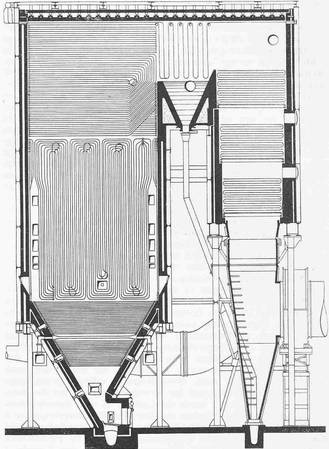
Abb. 4. Sulzer-Hochdruck-Einrohrkessel in Zweizug-Bauart mit Kohlenstaubfeuerung (Eckenbrenner) und Ljungström-Luftfritzer für 100 t/h Dampfleistung, 110 ata Betriebsdruck, 500° C Ueberhitzungstemperatur, Kesselhöhe 20 m. Masstab rd. 1 : 150
