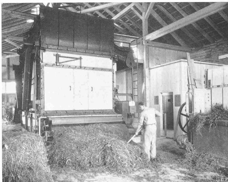
Abb. 3. Brown Boveri-Graströckner mit Wärmerückgewinnung, Modell 1942 der Landwirtschaftl. Genossenschaft Kiesen. — Wasserverdampfung 800 kg/h entsprechend 200 bis 400 kg/h Trockengras, je nach Wassergehalt im Frischgras
