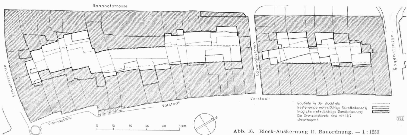
Abb. 16. Block-Auskernung lt. Bauordnung. — 1:1250
