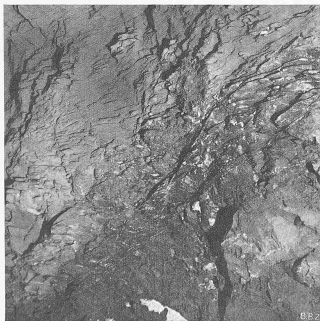
Abb. 8. Uebergang vom Kieselskalk (unten rechts) in die Drusbergschichten (oben links) bei Hm 1,375 Süd
