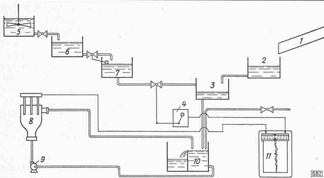
Abb. 7 (links). Schema einer Leeds & Northrup Antimon-Elektroden-Anlage in einer Papierfabrik. 1 Papier, 2 Sieb, 3 Mischbehälter, 4 Ventilbetätigung, 5 Alaunmischer, 6 Alaunbehälter, 7 Reguliergefäß, 8 Elektroden, 9 Pumpe, 10 Mischbehälter, 11 Registrier- und Regulierapparat
