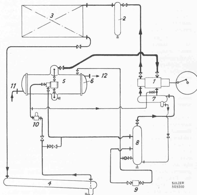
Abb. 1. Ammoniakleitungs-Schema der automat. Kühlanlage in Basel 1 Kompressor, 2 Oelabscheider, 3 Kondensator, 4 Akkumulierflasche, 5 Niveauregler, 6 Solekühler, 7 Receiver, 8 Absaugflasche, 9 Schwimmer, 10 Stoppventil, 11 von der internen Umwälzpumpe, 12 zum Sole-Akkumulator
