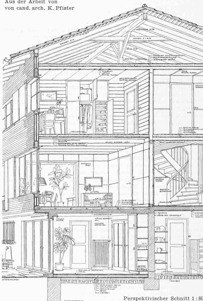
Perspektivischer Schnitt 1:80
