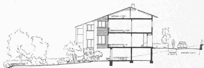
SCHNITT A-A M. 1:400
