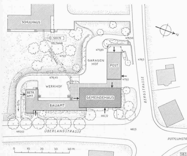
Abb. 1. Neue Gemeindefausthaus-Anlage in Zollikon (Zürich). — 1:1500
