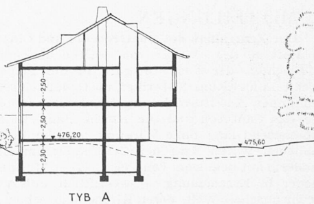
Siedlung an der Tachlisbrunnenstrasse, Winterthur. — Schnitt 1 : 350
