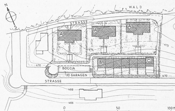
Lageplan der Siedlung 1 : 2000
