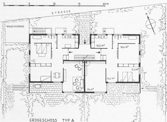
Zweifamilien-Doppelhäuser 1 : 350
