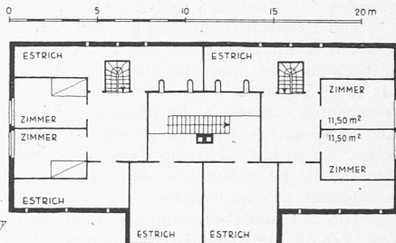
DACHGESCHOSS TYP A
