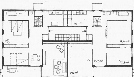
OBERGESCHOSS TYP A
