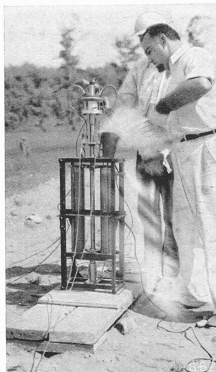
Abb. 3. Meteorolog. Höhenrakete
