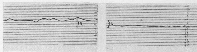
Abb. 12. Drehzahl-Zeitdiagramm. Links: Röhrenregler ausgeschaltet, Drehzahlsschwankungen, herrührend von Netzfrequenzschwankungen. Rechts: Nach Einschalten des Reglers Schwankungen der Drehzahl um den Mittelwert \pm 0,15\%
