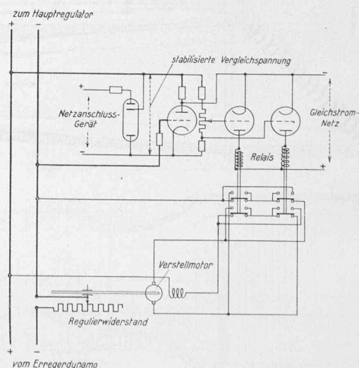
Abb. 11. Schema des Röhren-Spannungs- und Geschwindigkeitsreglers
