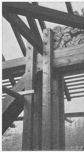
Abb. 7. Knotenpunkt II
