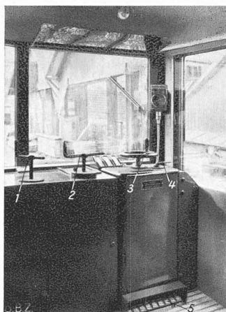
Abb. 5. Triebwagen-Führerstand. 1 Band-Klotzbremsen, 2 Klinkenbremsen, 3 Kontrolller, 4 Wende- u. Bremsumschalter, 5 Totmannpedal
