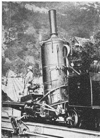
Abb. 1. Erste Zahnrad-Lokomotive der Rigibahn von 1871, gebaut von Ing. Niklaus Riggenbach in der S. C. B.-Werkstätte Olten
