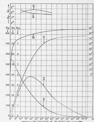
Fig. 17. Lentille C en régime de contre-pression égale au vide: Coeff. caract. en fonction de l'inclinaison \alpha de la lentille.
